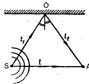
Hình 8.34 : Sơ đồ phát sinh tiếng dội S - nguồn âm ; A - người nghe ; SO ( l ) và OA ( l_2 ) - đường đi của âm phản xạ ; SA ( l ) - đường đi của âm trực tiếp.
