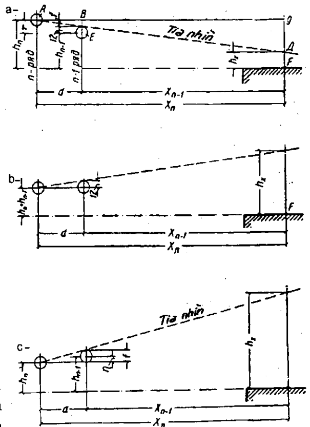
Hình 7.22 : Các sơ đồ kiểm tra điều kiện nhìn rõ a. Khi bố trí các hàng ghế có nâng cao ; b. Trên mặt phẳng nằm ngang ; c. Có độ dốc ngược.
