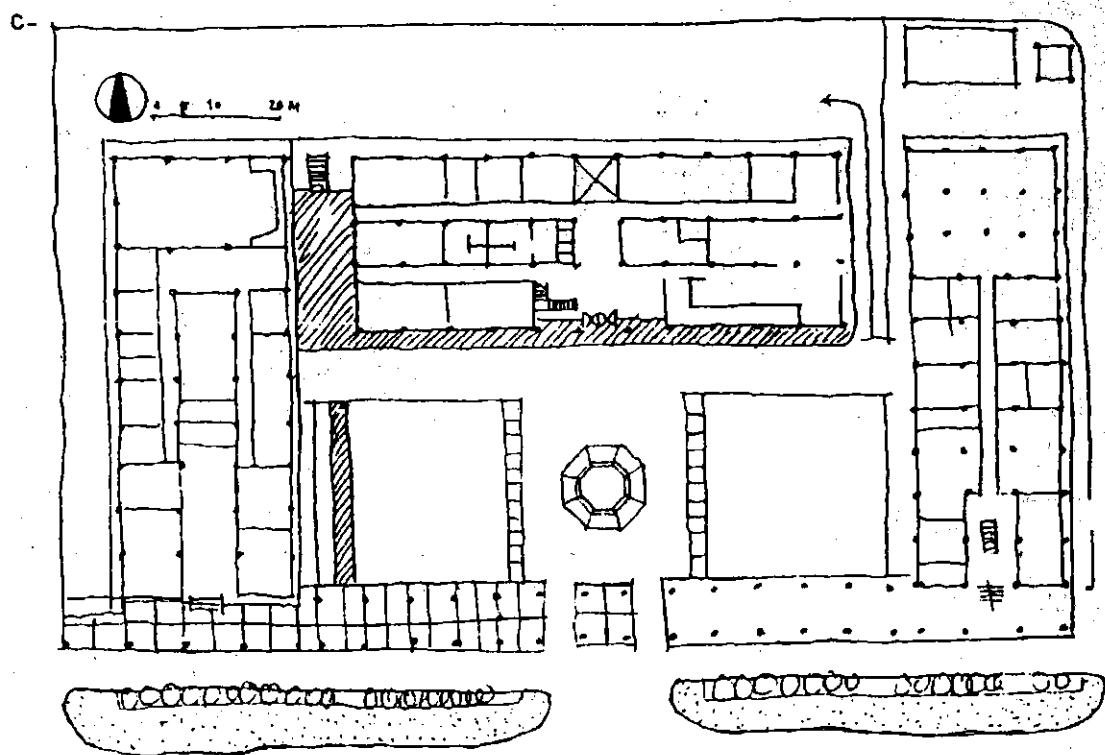
Hình 4.20 : Trụ sở tại Nhật a. Mặt đứng ; b. Mặt bên ; c. Mặt bằng.
