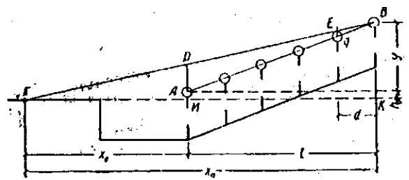
Hình 7.19 : Sơ đồ tính toán mặt cắt nâng cao các hàng ghế theo đường thẳng dốc.
