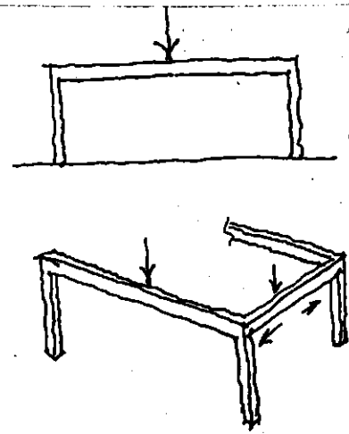
Hình 6.2 : Hệ khung - cột dầm
